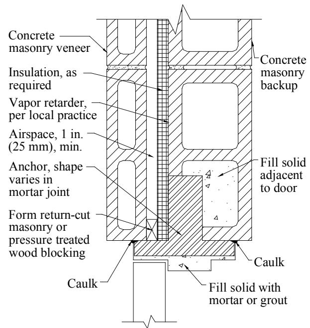
Figure 4—Metal Door Jamb
